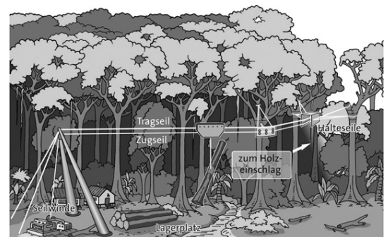
Die Baumschwebebahn: bodenschonender Holztransport
