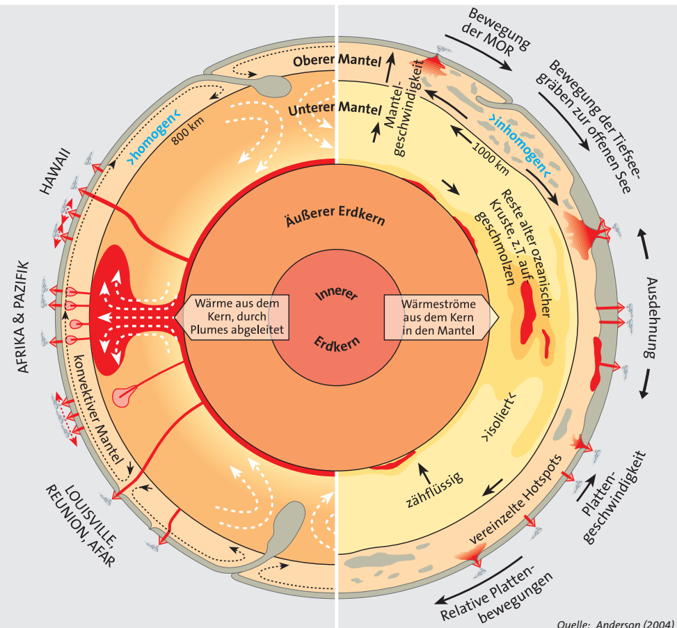
Plattentektonisches Modell mit Plumes (links) und ohne Plumes (rechts)
