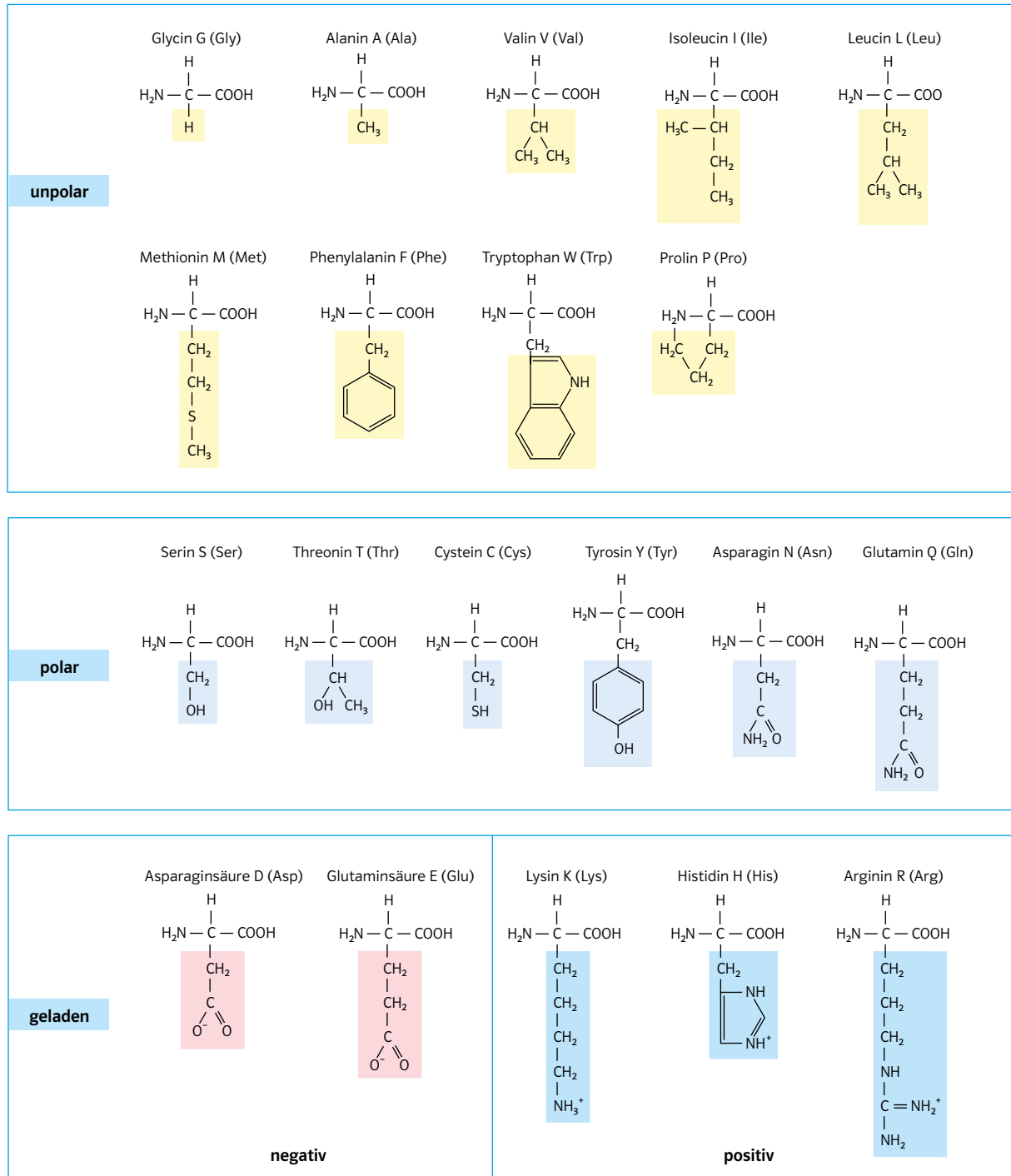
Strukturformeln der 20 Aminosäuren aus Proteinen mit dem Einbuchstaben- und dem Dreibuchstaben-Code als Abkürzung
