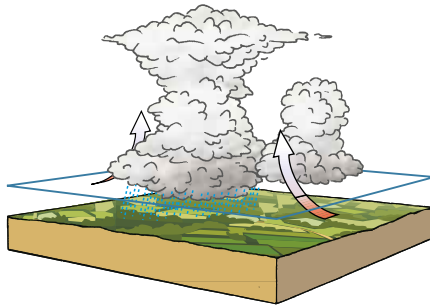
1 Konvektion
