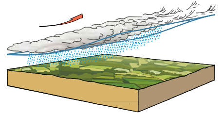
2 Advektion
