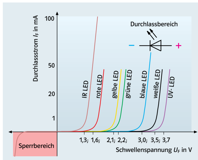
2 Kennlinien von Leuchtdioden
