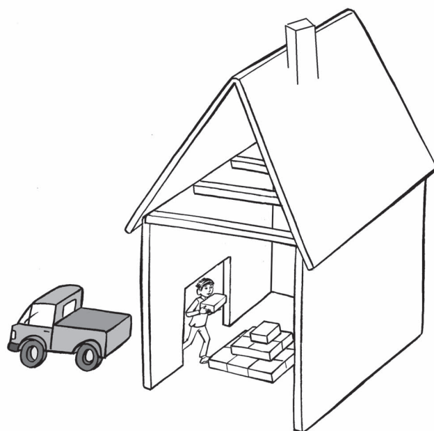
Lösung Problem 5: Eisblöcke zur Selbstmordhilfe
