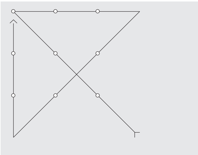
Lösung Problem 2: Verbindungslinie außerhalb des Punkte-Quadrates
