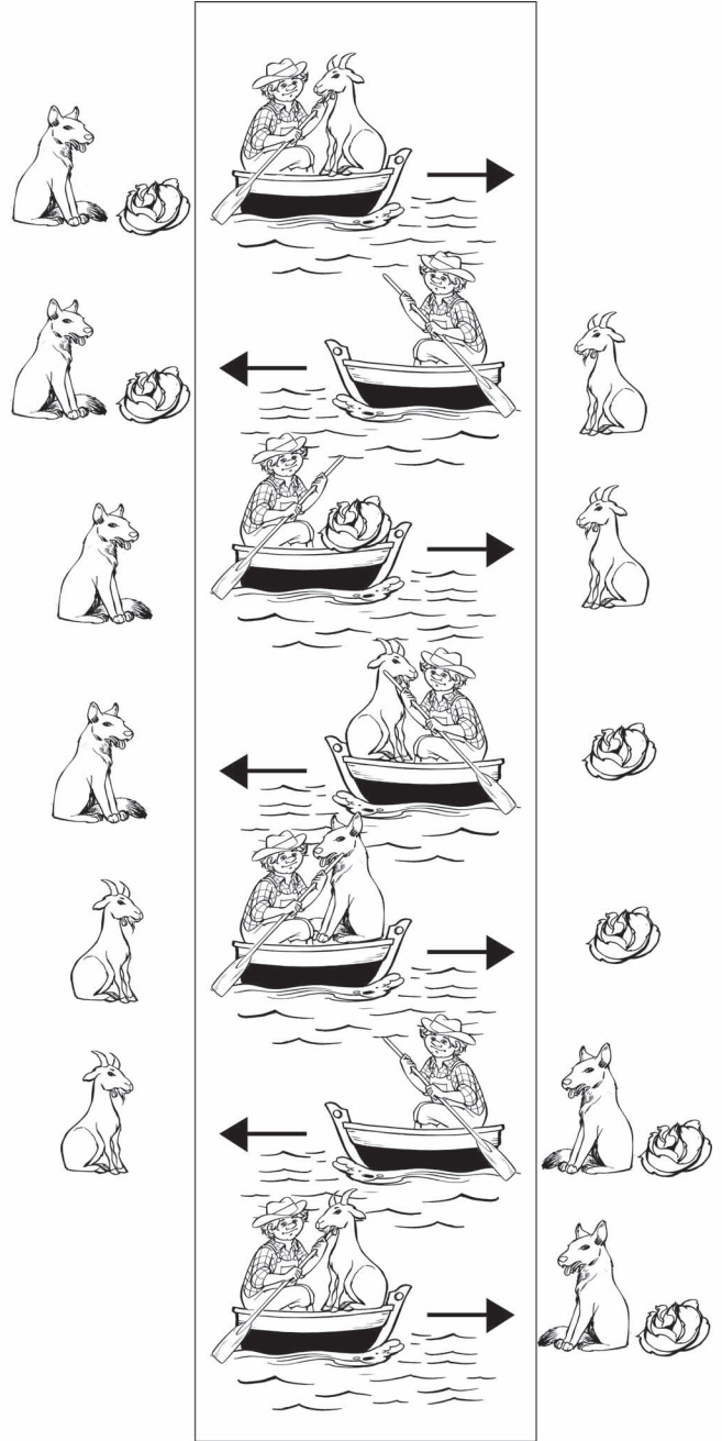
Lösung Problem 3: Die Ziege muss einmal zurückfahren
