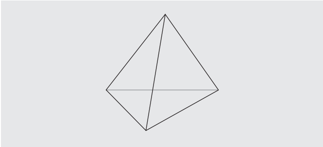
Lösung Problem 1: Ein Tetraeder Holzstäbchen
