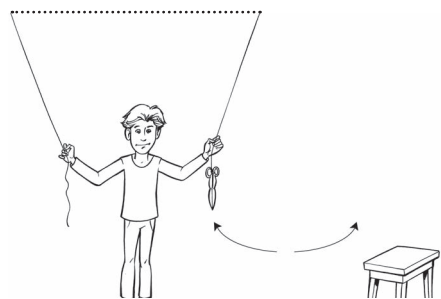
Lösung Problem 4: Scheren sind nicht nur zum Schneiden da
