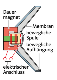
B5 Prinzip des elektrodynamischen Lautsprechers
