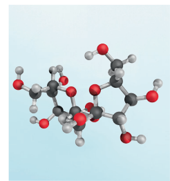
Zuckermolekülmodell
