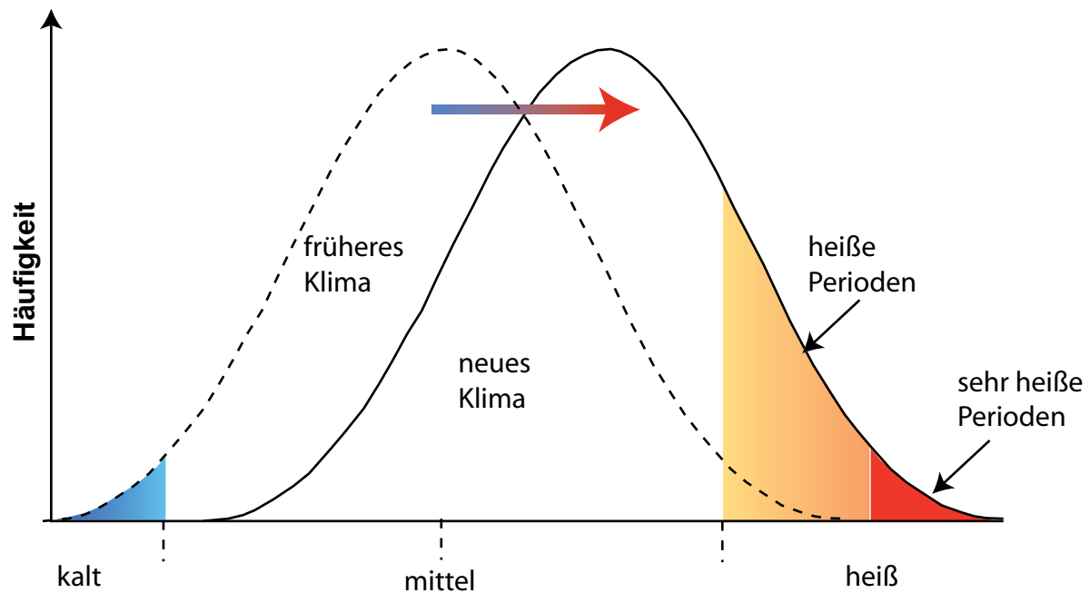
Abb.: Schematische Darstellung der Folgen einer Veränderung der mittleren Temperaturen auf die extremen Temperaturen. Quelle: nach IPCC [= Intergovernmental Panel of Climate Change] (2001)
