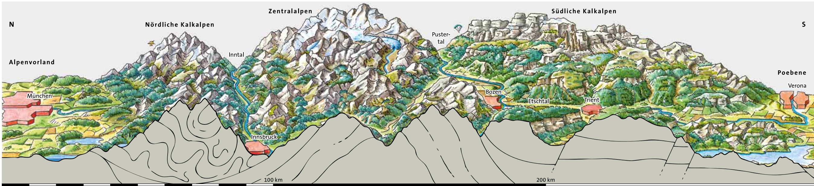
1 Querschnitt durch die Alpen
