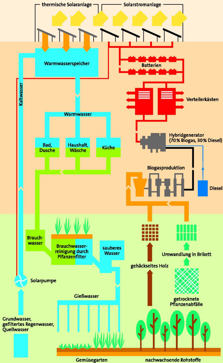
Schema autarke Energieversorgung für Gebäude auf dem Land | © Klett
